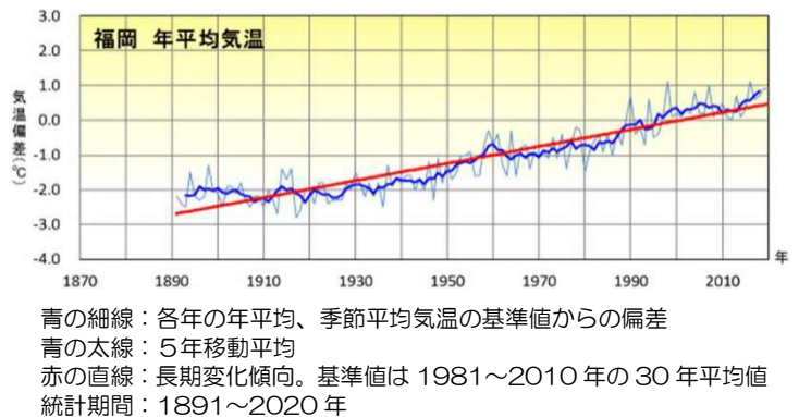
図3 年平均気温の経年変化
